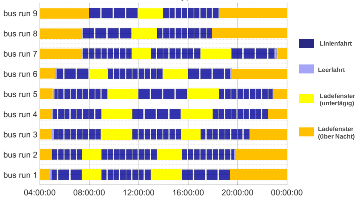
Abbildung 30: Betrieb mit Batteriebus 2, 150 kW Ladeleistung und vollelektrischer Heizung - Abstellhalle
