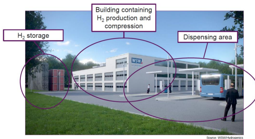
Abbildung 16: Wasserstofftankstelle mit Vor-Ort-Erzeugung mittels Elektrolyse für 200 bis 250 Busse [9]
