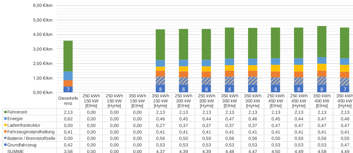
Abbildung 41: Batteriebusse mit Ladung am Rendezvous-Platz - Annuitäten in Euro pro Nutzkilometer (ohne Förderung)
