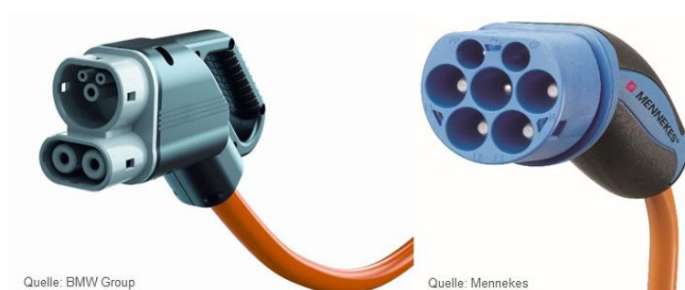
Abbildung 8: Konduktives Laden via Plug-In (Combo-2 & Typ-2 Stecker)
