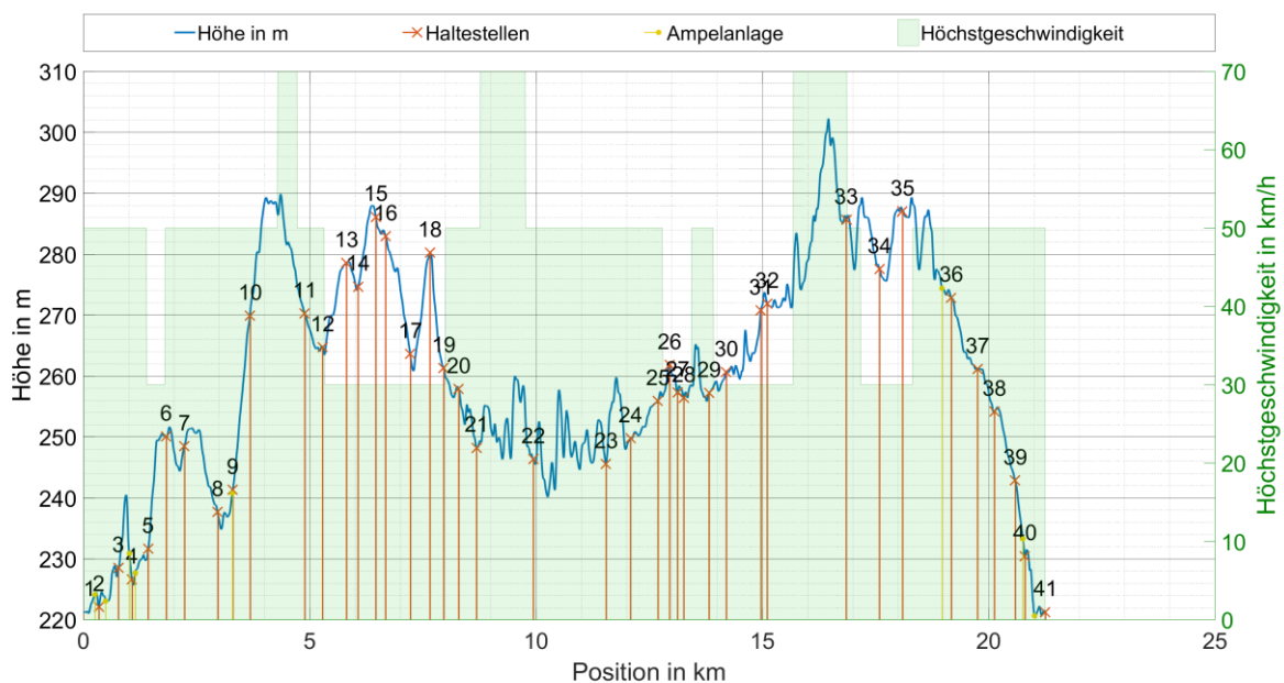
Abbildung 19: Höhenprofil der Linie 525
