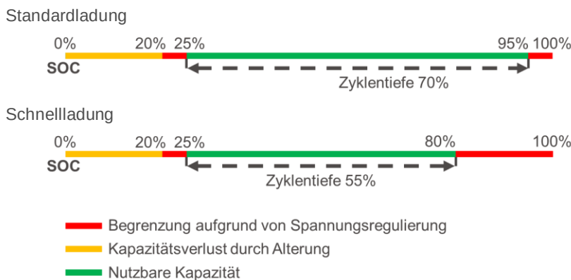
Abbildung 6: Beispiel für zulässige Betriebsbereiche der Batterie bei Schnell- und Standardladung
