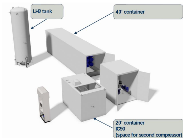
Abbildung 15: Schematische Darstellung einer Wasserstofftankstelle für 10 Busse [6]
