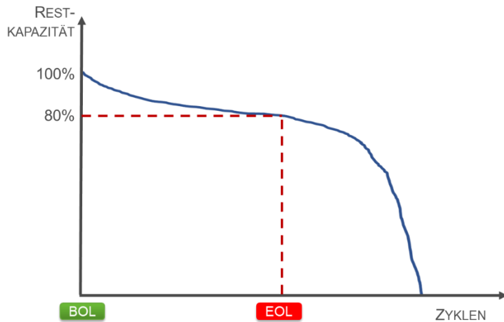
Abbildung 5: Exemplarischer Kapazitätsverlust einer Batteriezelle bedingt durch Alterung
