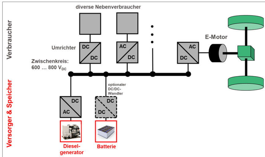
Abbildung 10: Antriebstopologie des seriellen Hybridbusses
