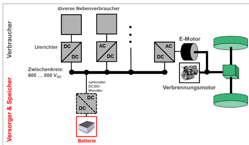
Abbildung 11: Antriebstopologie des parallelen Hybridbusses
