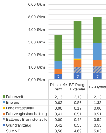
Abbildung 42: Brennstoffzellenbusse - Annuitäten in Euro pro Nutzkilometer (ohne Förderung)
