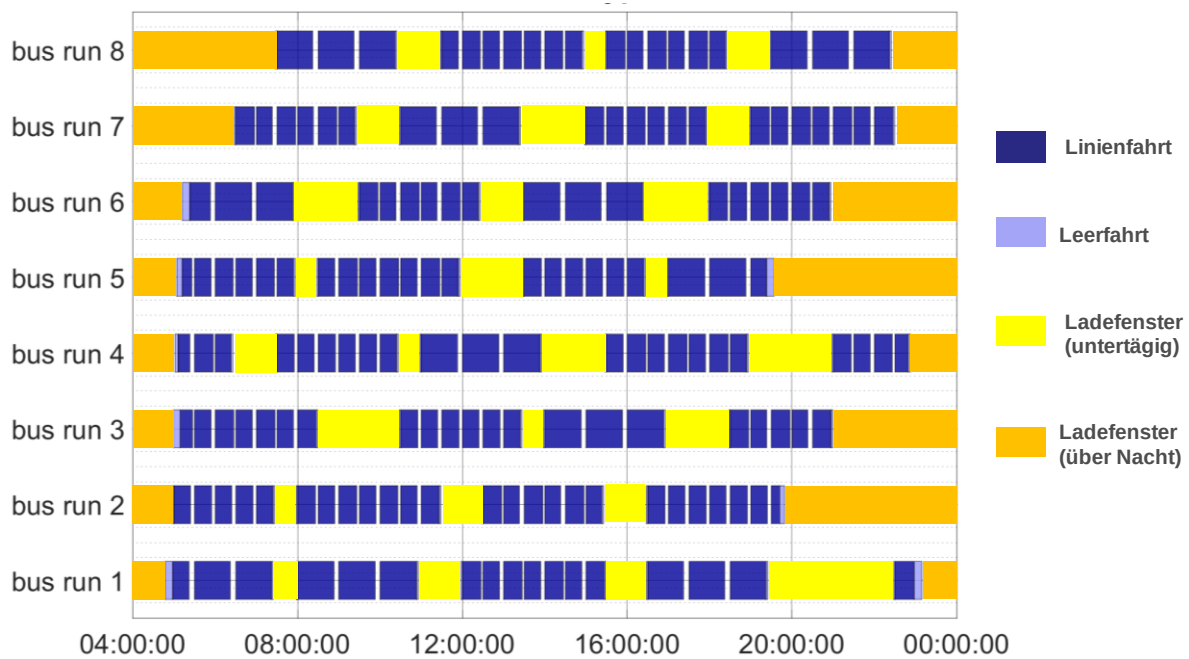
Abbildung 34: Betrieb mit Batteriebus 1, 450 kW Ladeleistung und Hybridheizung - Abstellhalle
