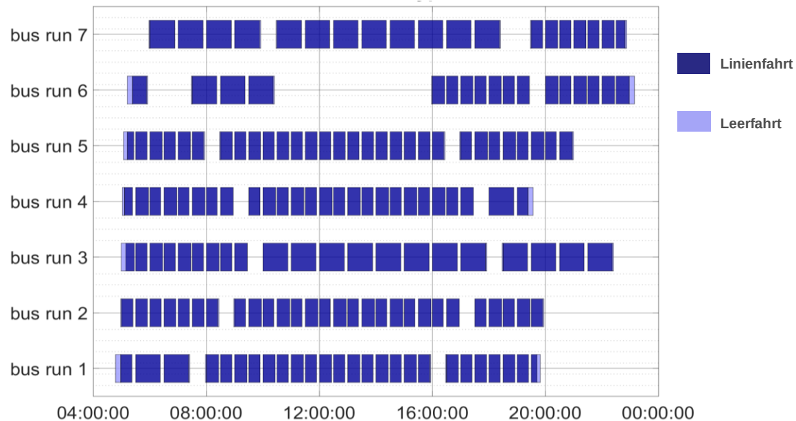
Abbildung 29: Einsatzkonzept Dieselbusse
