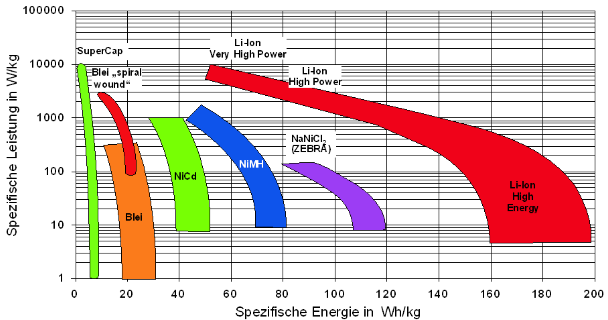
Abbildung 4: Ragone-Diagramm aktueller Batterietechnologien
