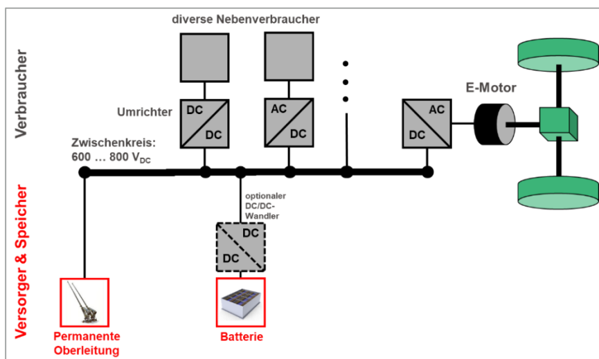
Abbildung 13: Antriebstopologie des batteriebetriebenen Oberleitungsbusses
