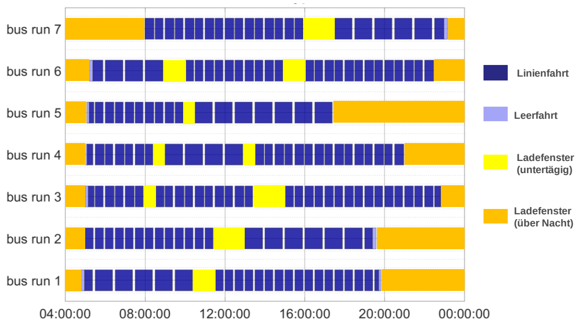
Abbildung 36: Betrieb mit Batteriebus 3, 450 kW Ladeleistung und Hybridheizung - Rendezvous-Platz
