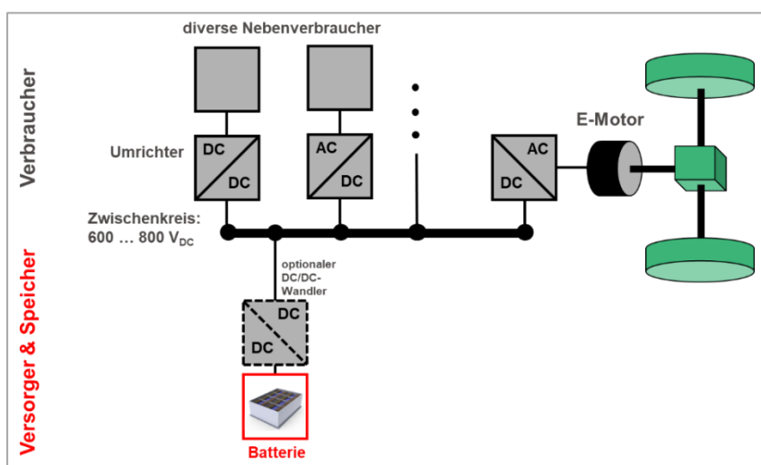
Abbildung 7: Antriebstopologie des Batteriebusses
