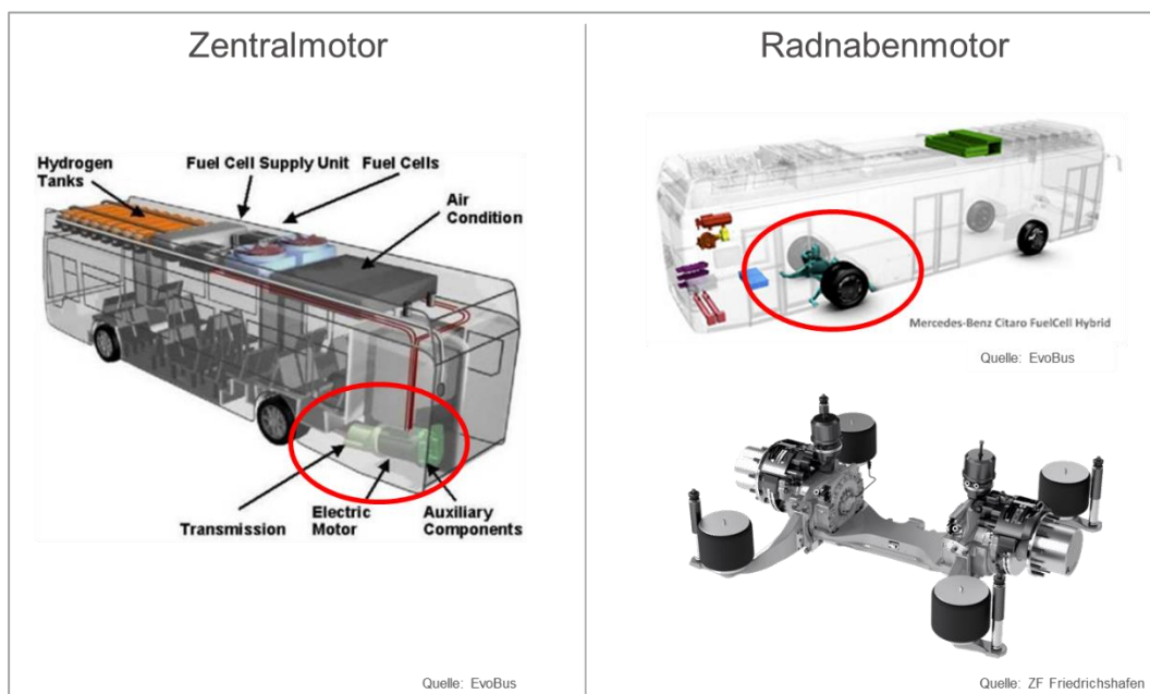
Abbildung 2: Zentralmotor vs. Radnabenmotor
