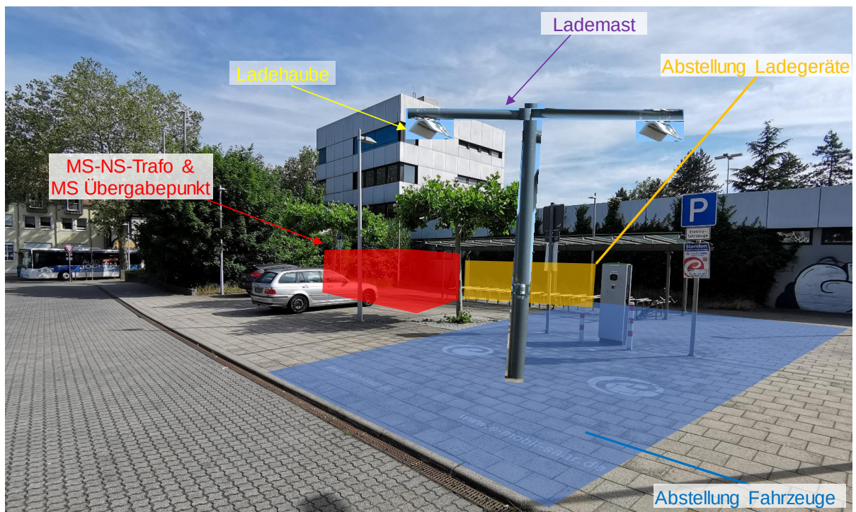
Abbildung 27: Aufstellungskonzept Rendezvous-Platz mit Schnellladung und Lademast
