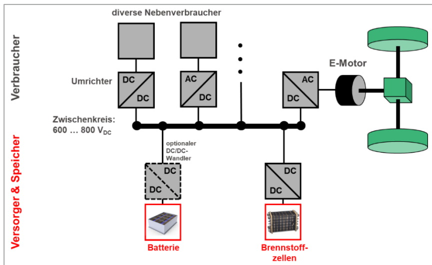
Abbildung 14: Antriebstopologie des Brennstoffzellenbusses
